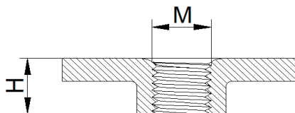
Durchgangsloch mit Durchzug
