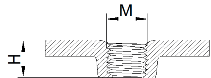
Sackloch
