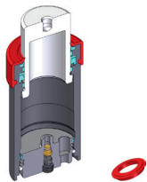
Standard+Abstreifring NV 5 NCS50-25-A-W
